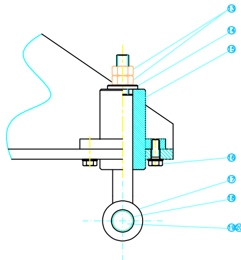
DETALLE ARTICULACION FONDO (E1:2.5)
