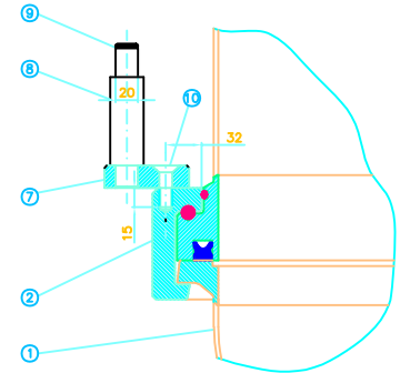
DETALLE FIJACION CILINDRO BAYONETA (E1:2.5)
