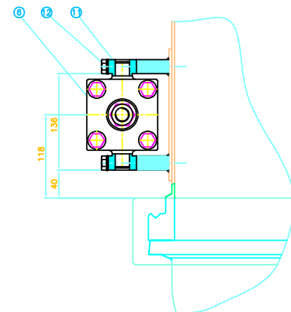
DETALLE FIJACION CILINDRO BAYONETA (E1:2.5)
